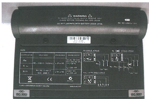
Рисунок 2 - Внешний вид тестеров заземления Fluke 1623-2 и Fluke 1625-2, вид снизу.
