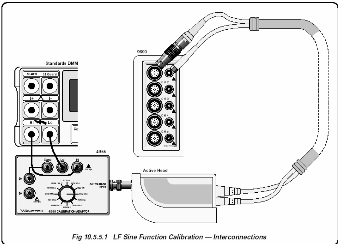
Рис. 10.5.5.1. Калибровка функции «LF Sine» - межсоединения
