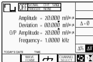
Рис. 4.4.8 Девиация выбрана как ΔV
