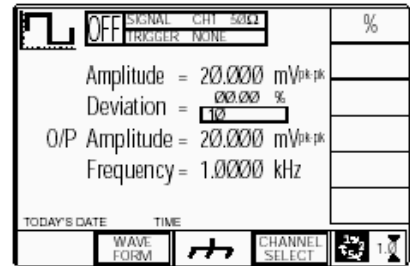
Рис. 4.4.6 Ввод числа — изменение величины отклонения и обозначение экранных кнопок
