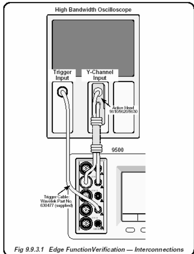
Рис. 9.9.3.1. Поверка функции фронта - межсоединения
