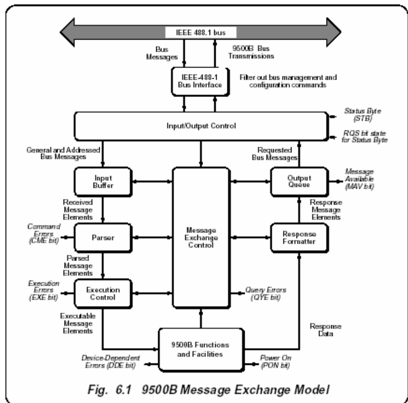
Рис.6.1. Модель обмена сообщениями
