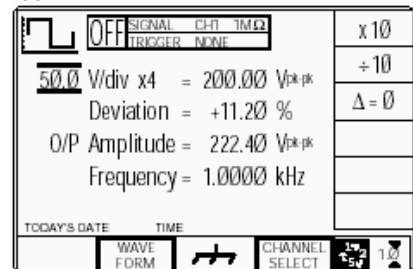
Рис. 4.4.12 Переход в режим Scope
